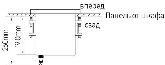
Схема установки
