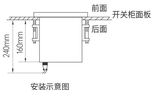
HKC-3D 智能监控装置安装尺寸及安装示意图
