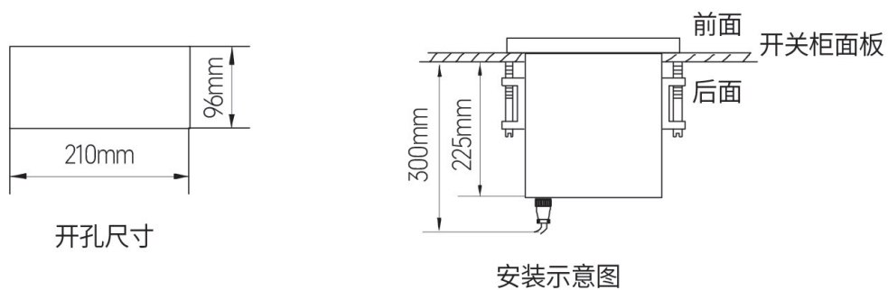
图6 YK-3 控制器安装尺寸及安装示意图
