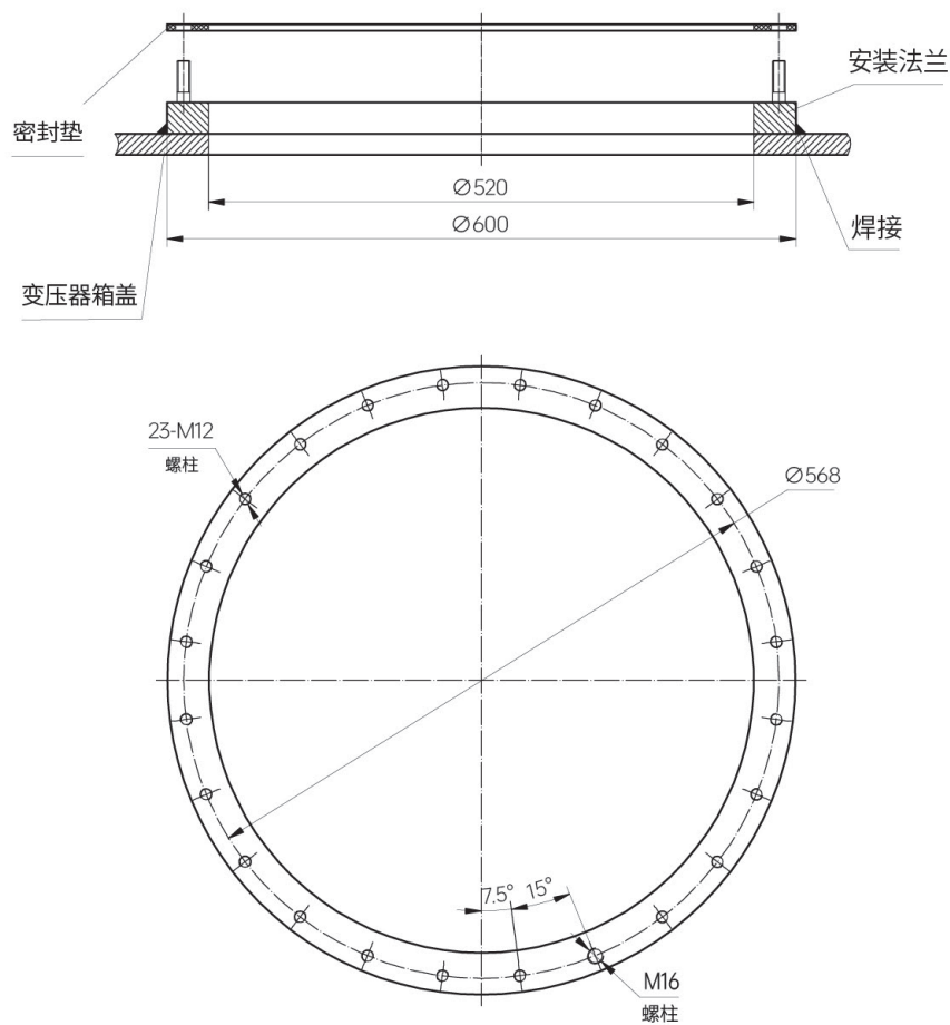
图5 SY有载分接开关安装法兰及箱盖开控尺寸图
